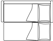
Divano letto da 216 L. 216 P. 100 H. 75 materasso sopra 89x194 H. 15 materasso sotto 75x186 H. 15
