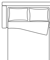
Laterale letto da 182 dx/sx L. 182 P. 103 H. 87 materasso 140x195 H. 12
