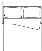
Divano letto da 184 L. 184 P. 98 H. 88 materasso 160x195 H. 18
