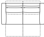
divano da 200 con 2 relax L. 200 P. 101/164 H. 98
