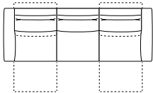
divano da 280 con 2 relax L. 280 P. 101/164 H. 98
