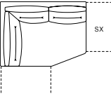
angolare da 162x122 dx/sx L. 162 P. 122 H. 88
