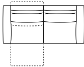
divano da 220 con 1 relax dx/sx L. 220 P. 101/164 H. 98
