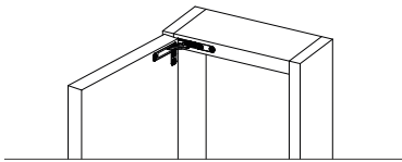
DETTAGLIO CERNIERA AIR / AIR HINGE DETAIL
