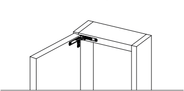
DETTAGLIO CERNIERA AIR / AIR HINGE DETAIL
