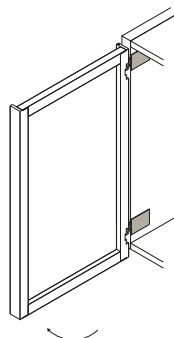
DETTAGLIO CERNIERA / HINGE DETAIL
